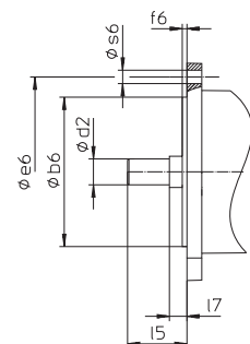
Abb. Motorabtrieb Picture: Motor output Figure: Sortie de moteur
