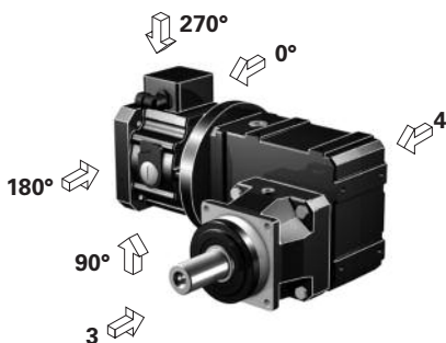
Motoradapter mit Bremse MB Motor adapter with brake MB Lanterne pour moteur avec frein MB
